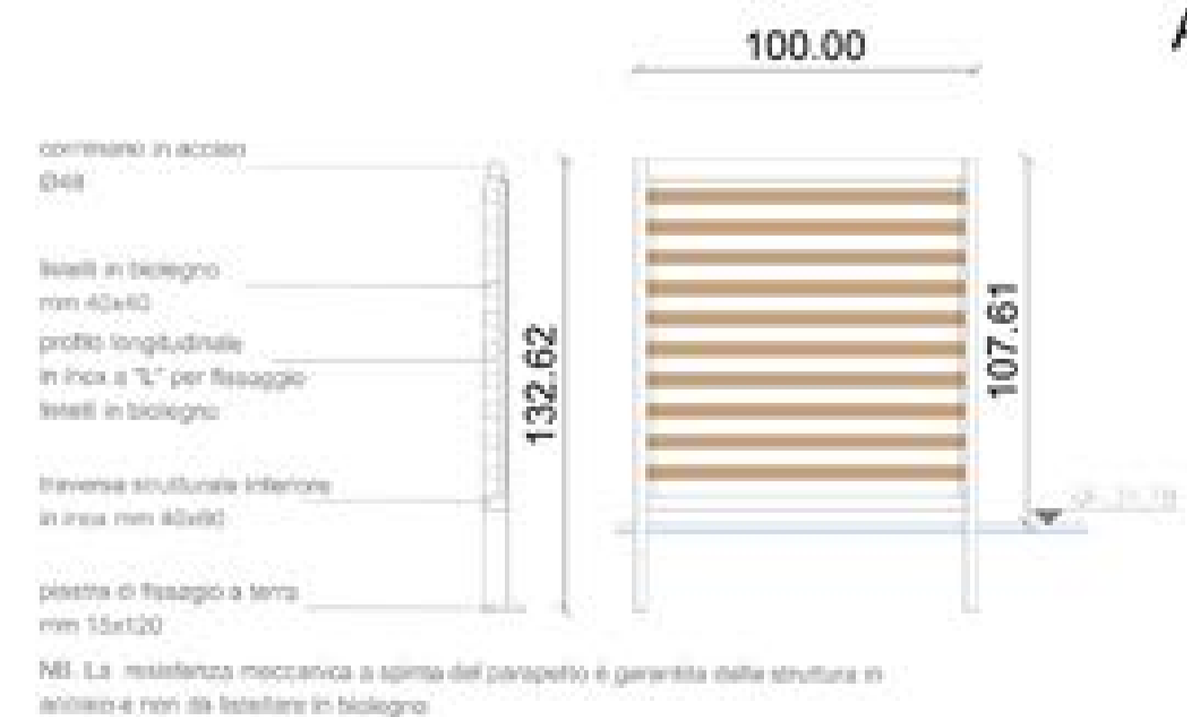
DETTAGLIO PARAPETTO Scala 1.20
