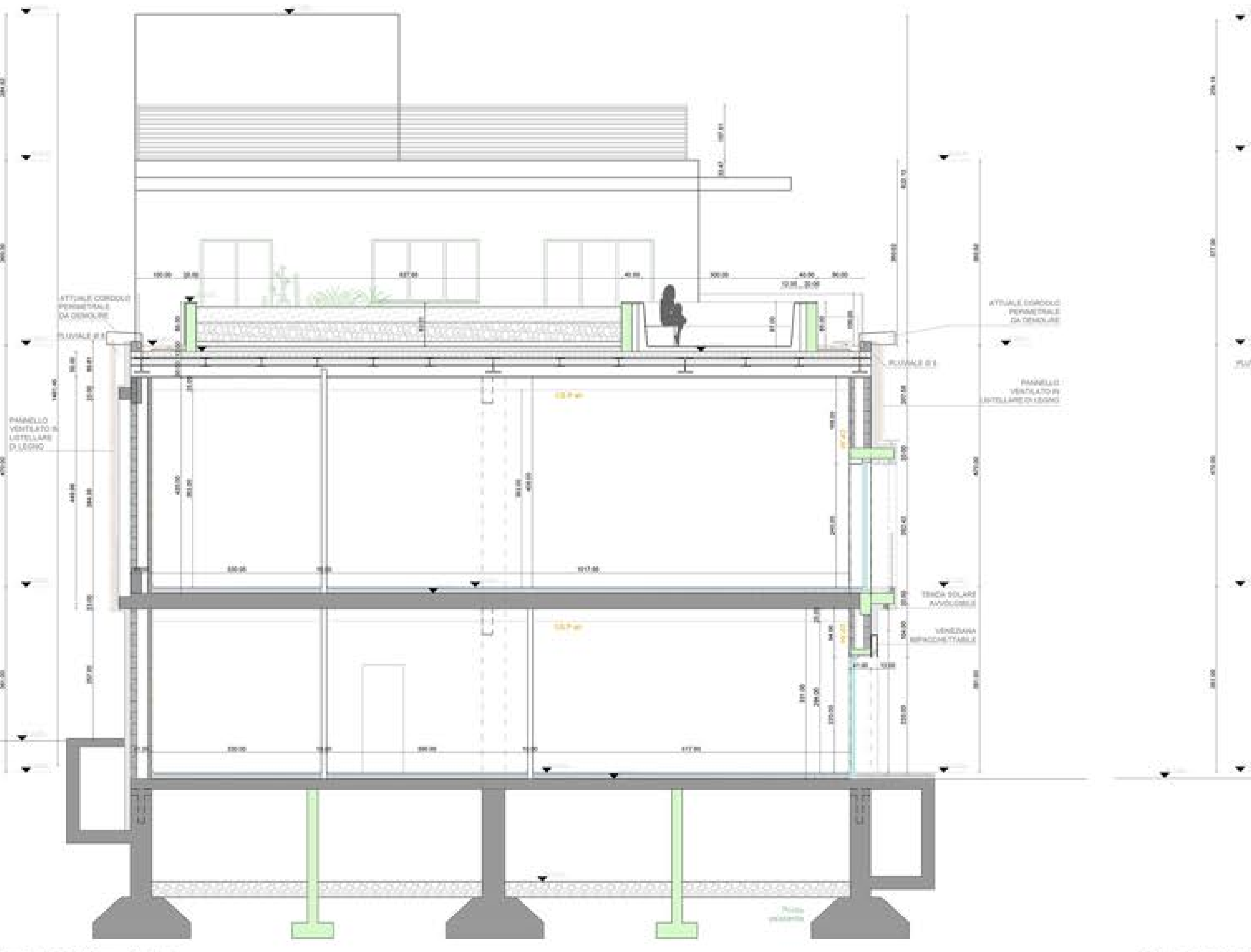
SEZIONE AA'
