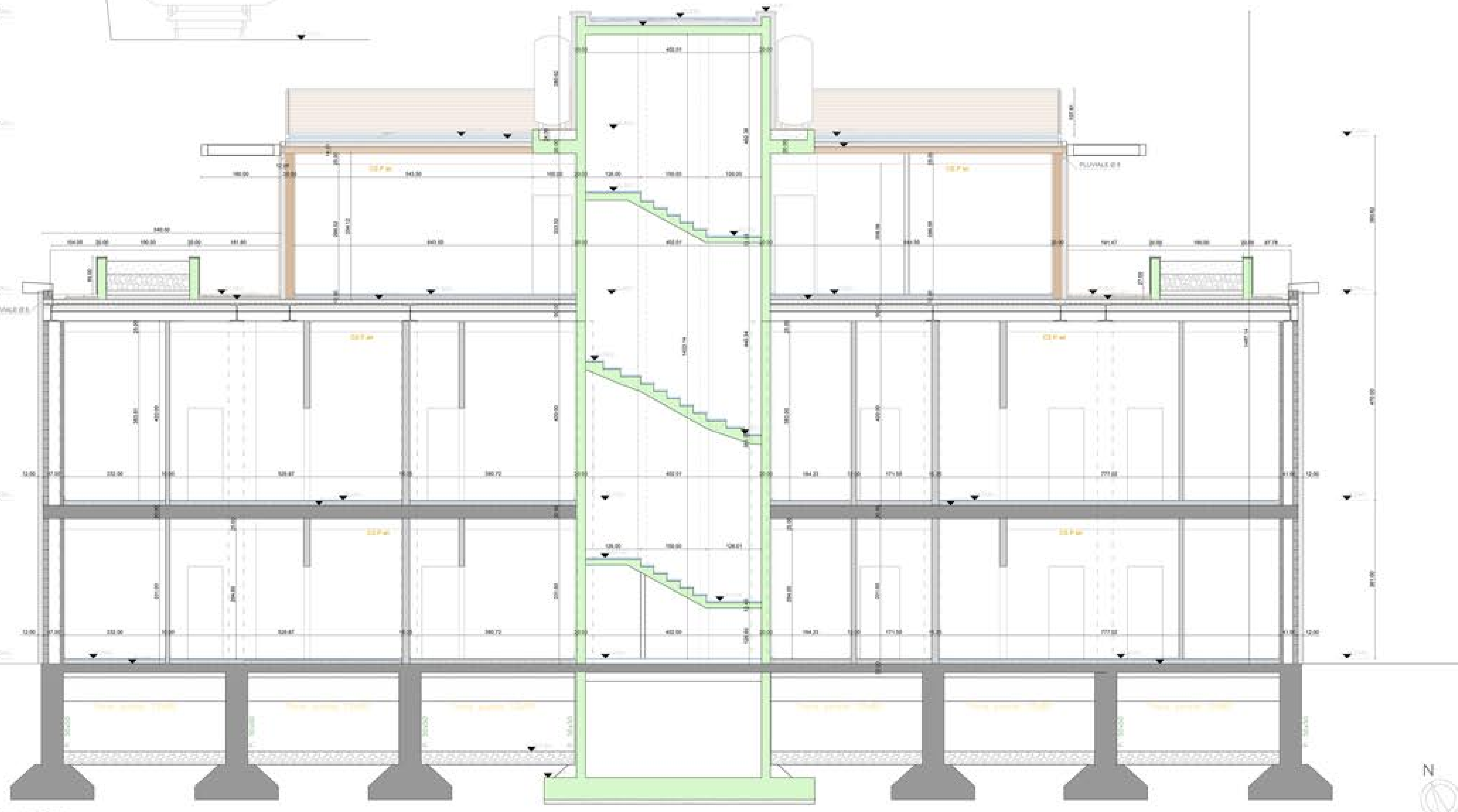
SEZIONE EE'
