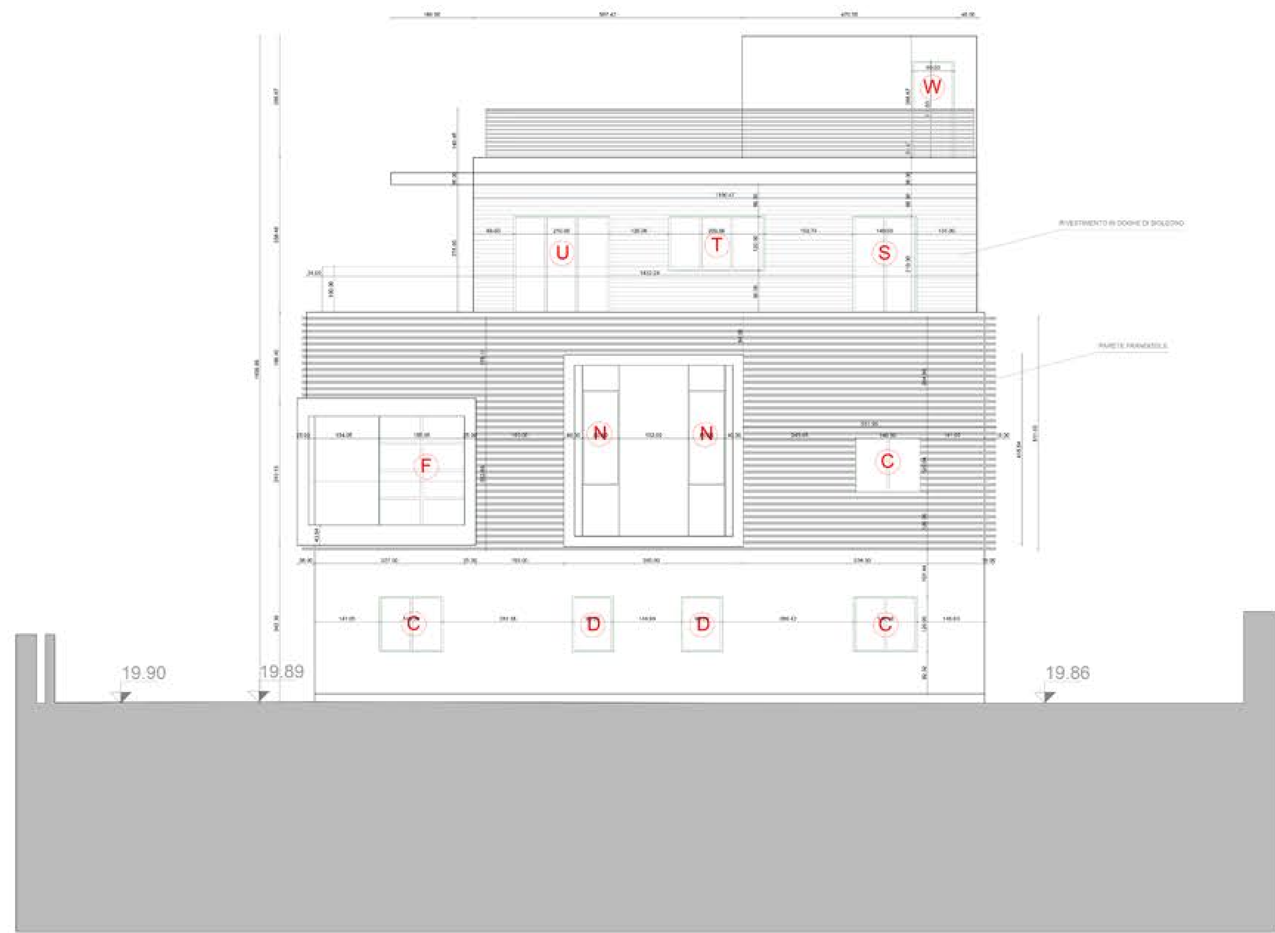
PROSPETTO EST
