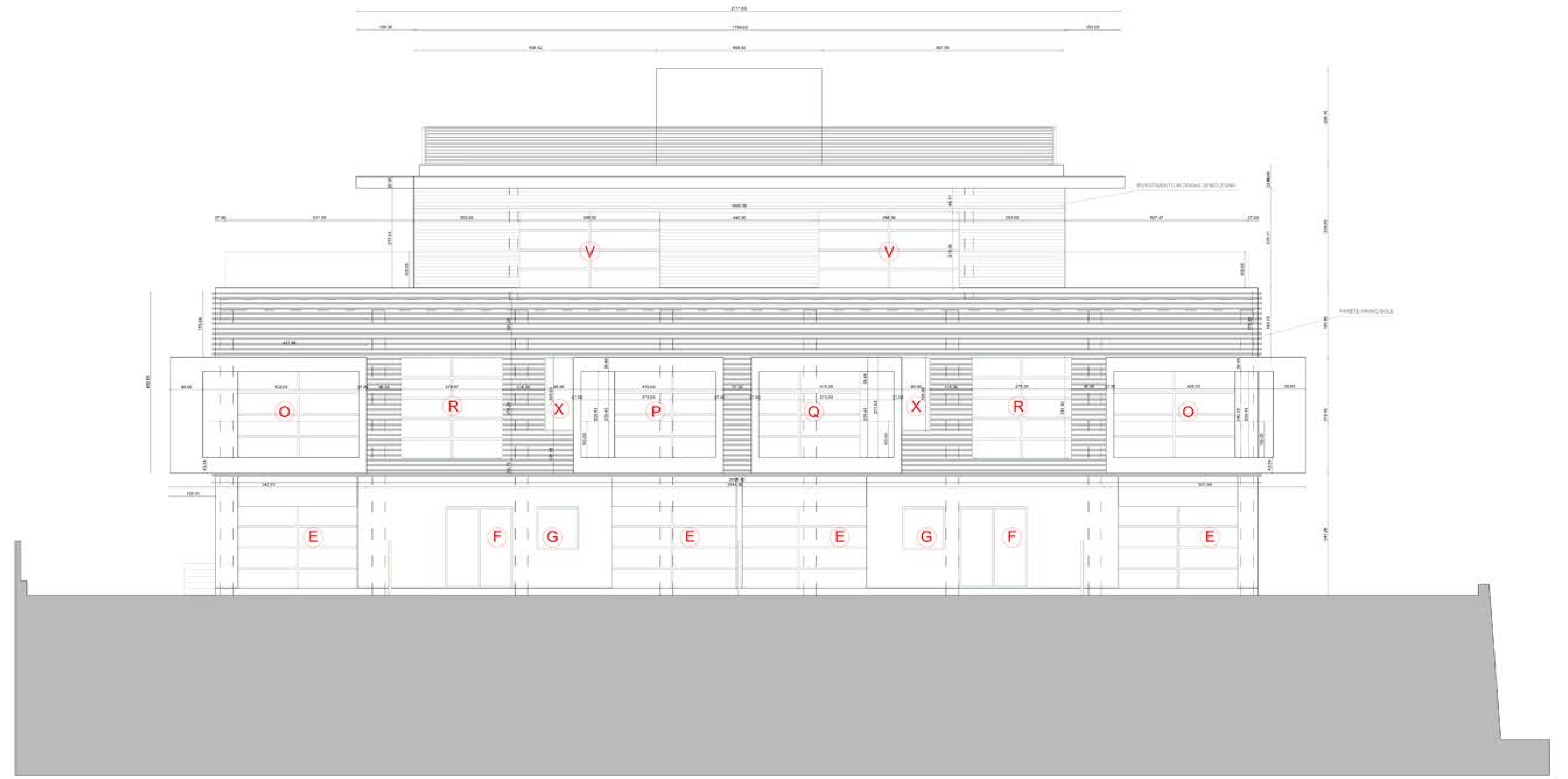
PROSPETTO SUD
